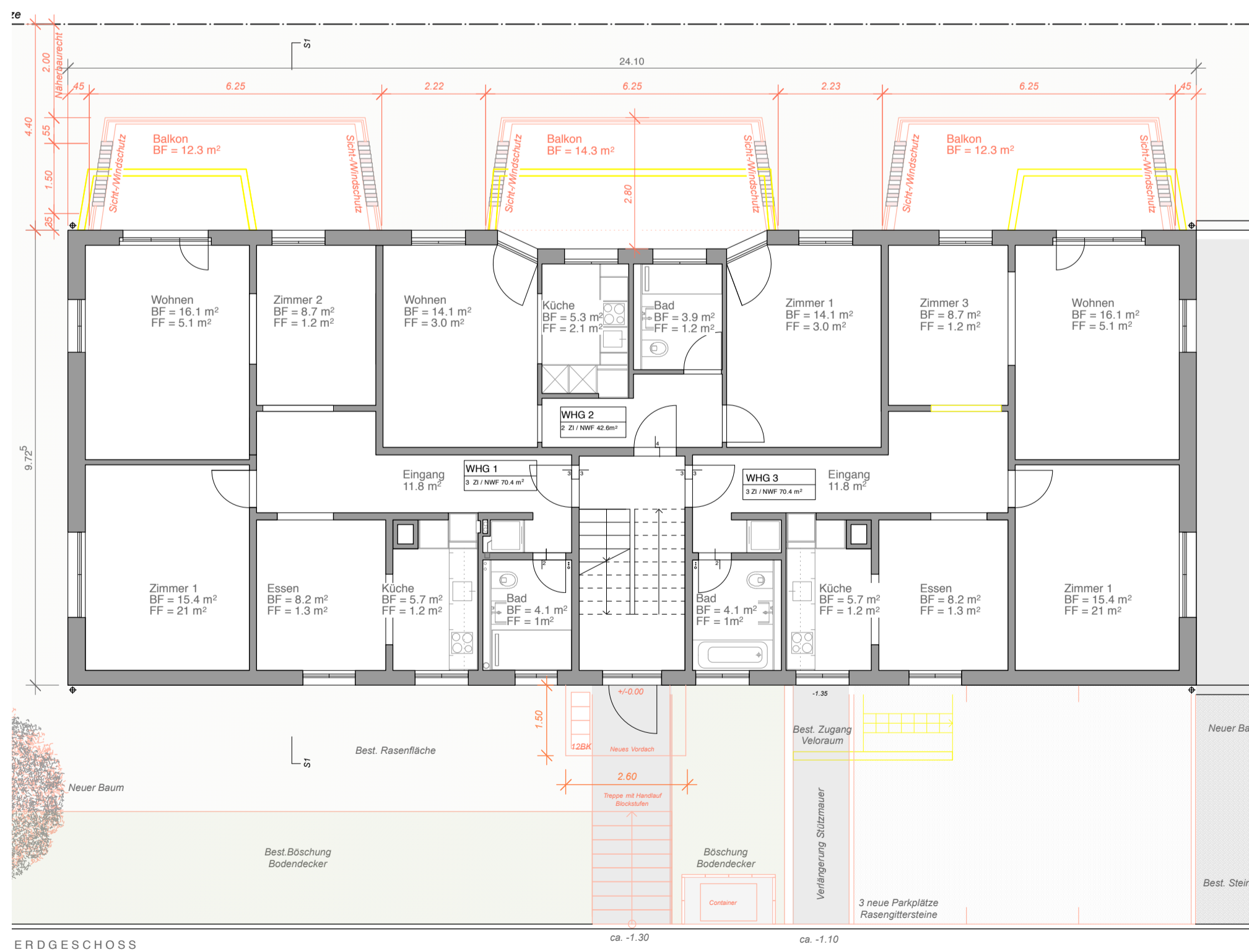
ERDGESCHOSS
